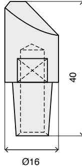
\varnothing 16 12411
