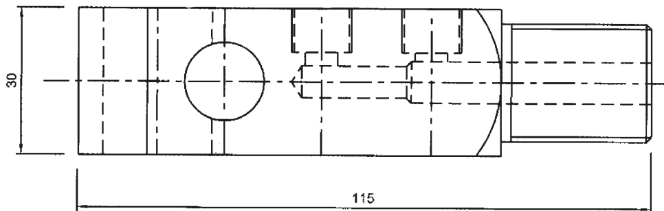
TEB8-SD superiore diritta
